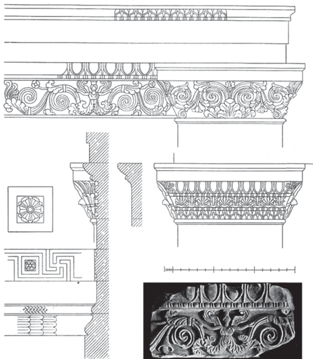
2 Wandaufbau des Pterons im Artemision von Magnesia am Mäander
