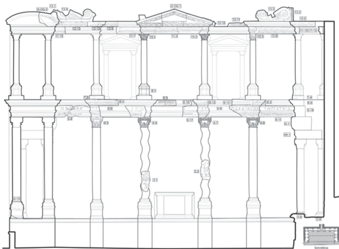
2 Steingerechte Rekonstruktion des Nymphaeum Traiani von U. Quatember
