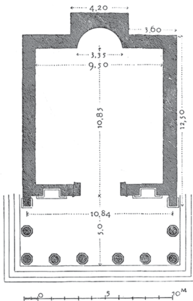
1 Termessos, sog. Tempel N1 (Lanckoroński 1892)
