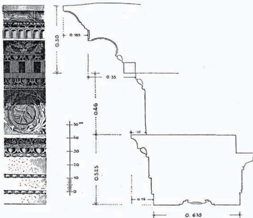
1 Gebäk der Celsusbibliothek, Untergeschoss
