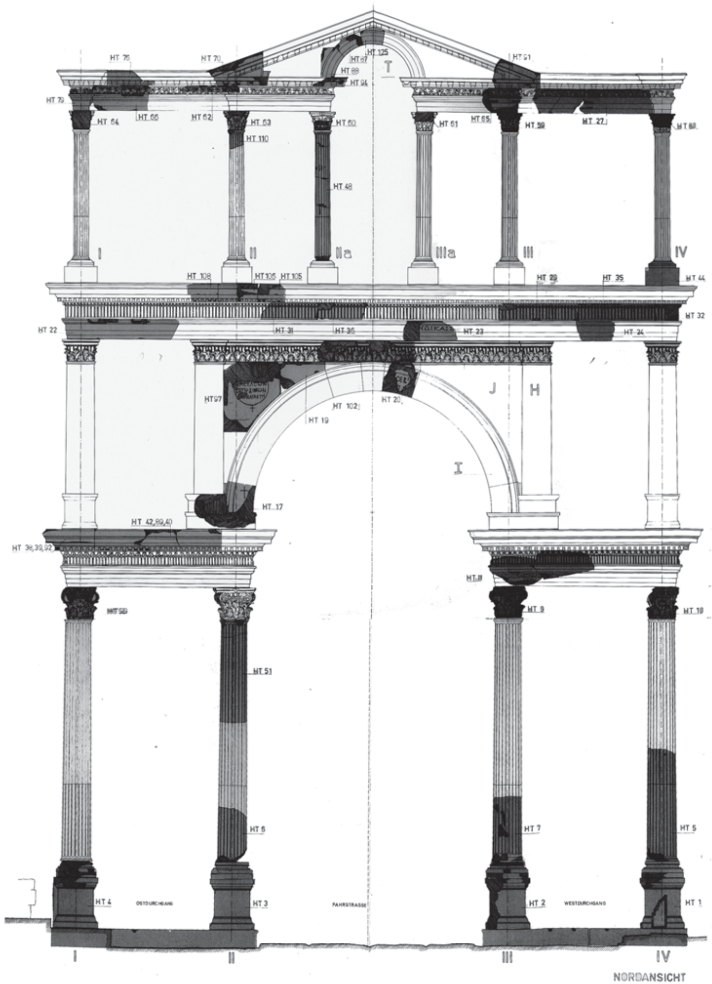
Steingerechte Rekonstruktion des »Hadrianstors« von H. Thür
