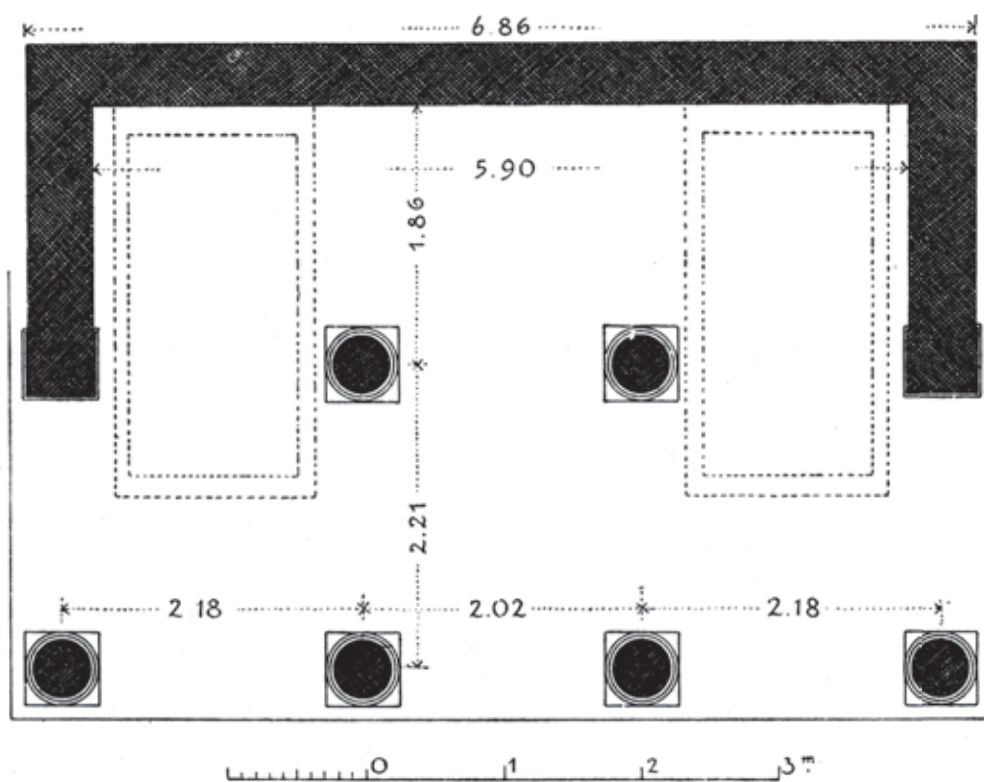
2 Termessos, Grabbau der Aurelia Padamuriane Nanelis (Heberdey – Wilberg 1900)
