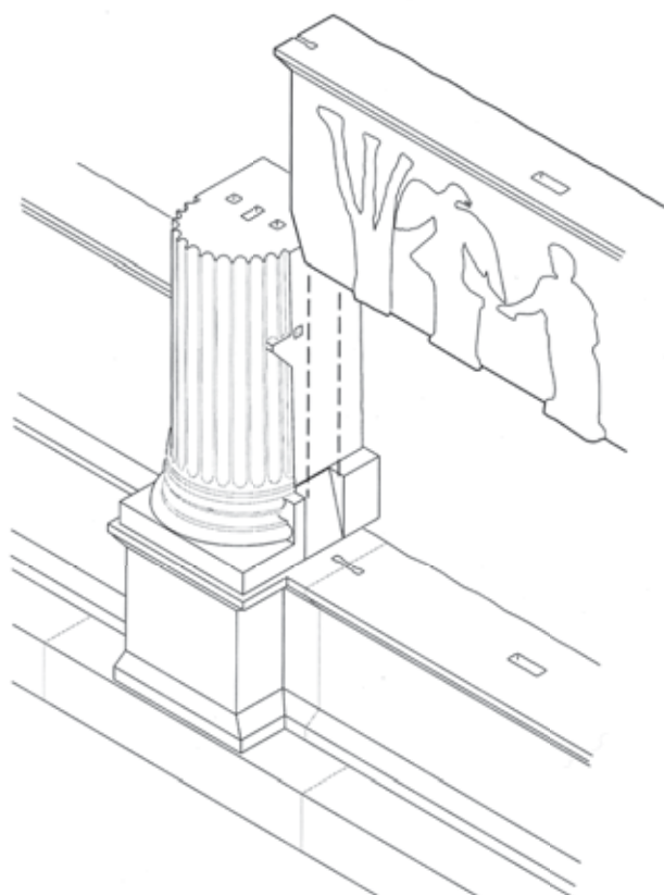
2 Aphrodisias, Basilika. Wechselseitige Bezugnahme von Reliefs und Architektur (Stinson 2008b)
